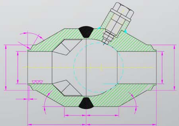
球 閥
